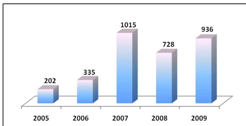
Р и с у н о к 2 М и г р а ц и о н н ы й п р и р о с т н а с е л е н и я р е с п у б л и к и со странами СНГ и Балтии (человек)
