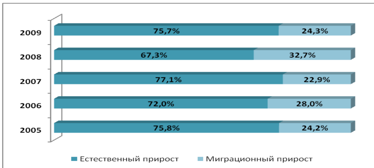
Р и с у н о к 1 Доля естественной и миграционной убыли в общей убыли населения (в процентах)
